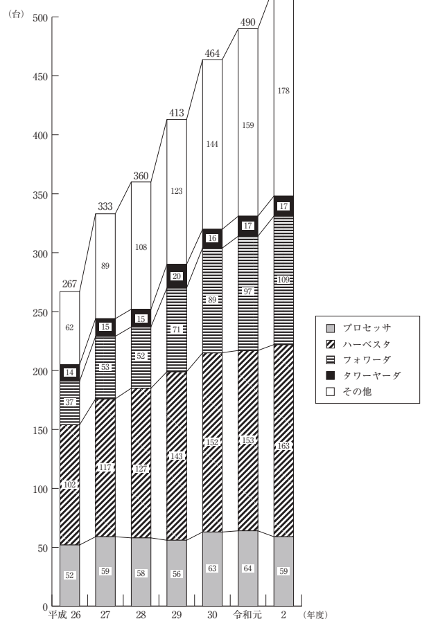
高性能林業機械の保有状況
